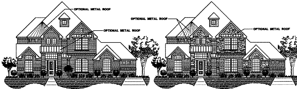
ELEVATION 'B'
